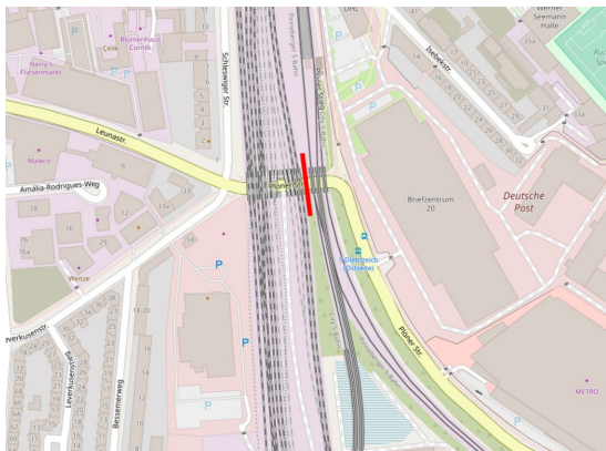
An der Eisenbahnbrücke über die Plöner Straße ist der Einbau einer Kabelhilfsbrücke geplant
